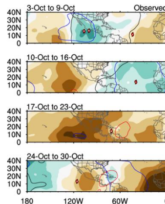
Comportamiento de la MJO en octubre
